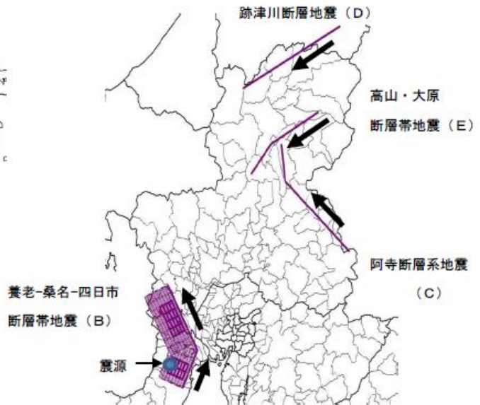
内陸直下型地震の断層の位置図
